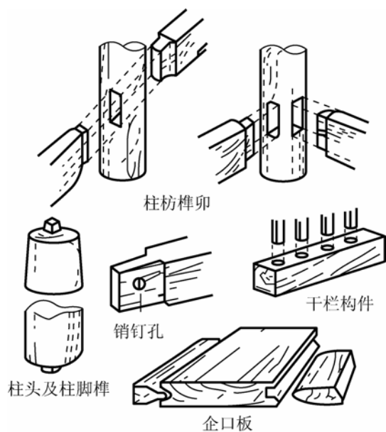
图 1.10 河姆渡遗址出土的榫卯类型
