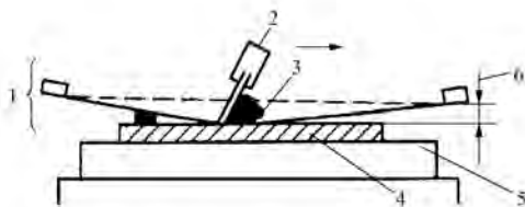
图 1-4 平型丝网印刷机印刷部的构成
