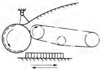
图 1-6 圆压平型印刷机
