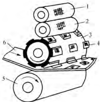
图 1-1 凸版印刷机印刷部的构成
