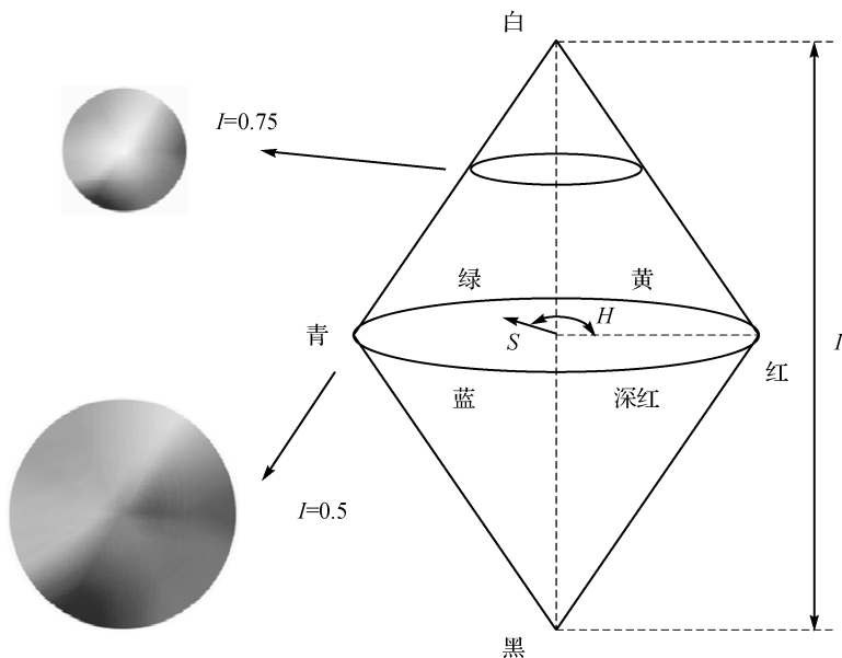
图 1.6 HSI 颜色模型
