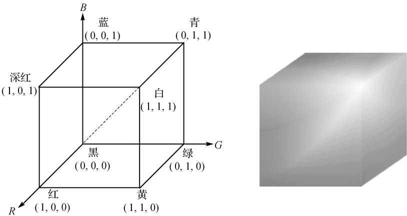
图 1.2 RGB 立方体
