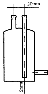
图 2 贮气瓶
