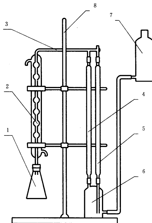
1—锥型瓶(5.1.3);2—冷凝管(5.1.4);3—三通活塞(5.1.5);4—量气管(5.1.6); 5—参比管(5.1.6);6—贮气瓶(5.1.7);7—水准瓶(5.1.8);8—支架
