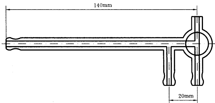
图 1 三通活塞
