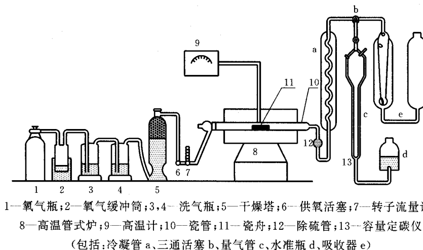
图 1 测量装置
