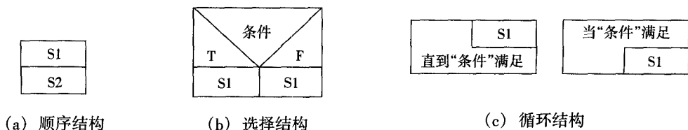
图 1-4 N-S 图的三种基本控制结构
