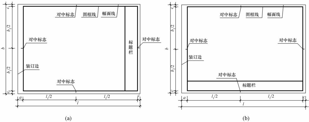
图 1-1 A0~A3 横式幅面
