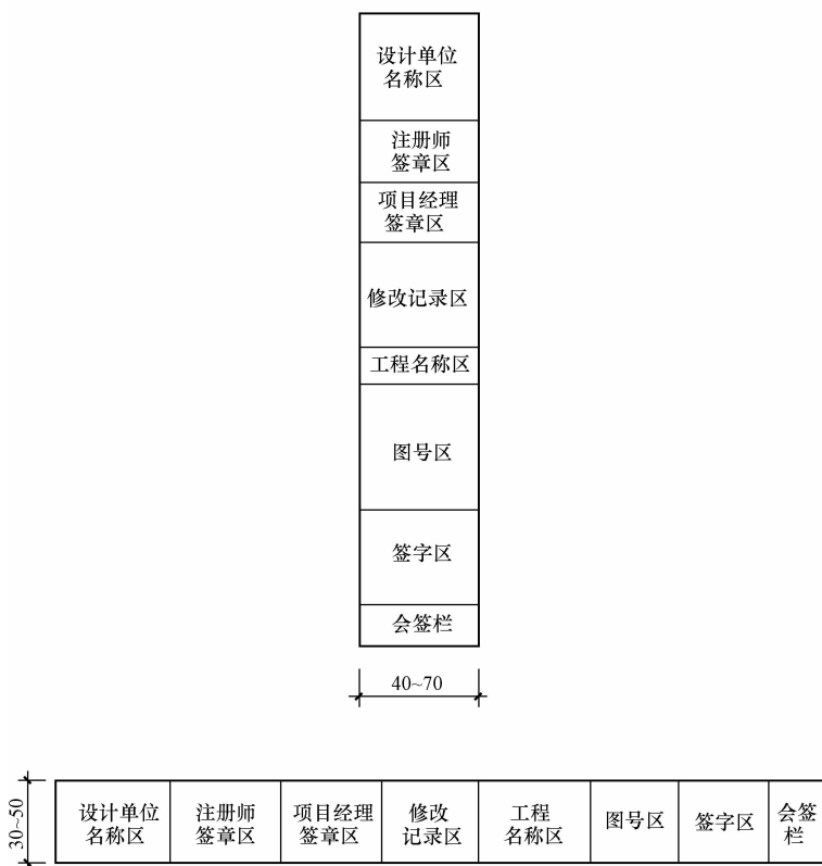
图 1-3 标题栏
