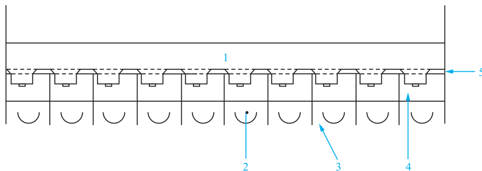
1. 工作台 2. 评价小间 3. 隔板 4. 小窗 5. 开有样品传递窗口的隔板
