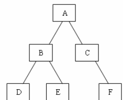
图 1-1 族谱二叉树
