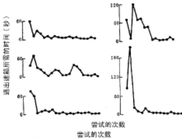
图1-2 桑代克迷箱实验5只猫的学习曲线
