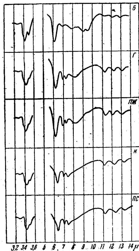
图 4. 一系列苏联煤的红外吸收光谱 (根据 О. И. Зильбербранд)
