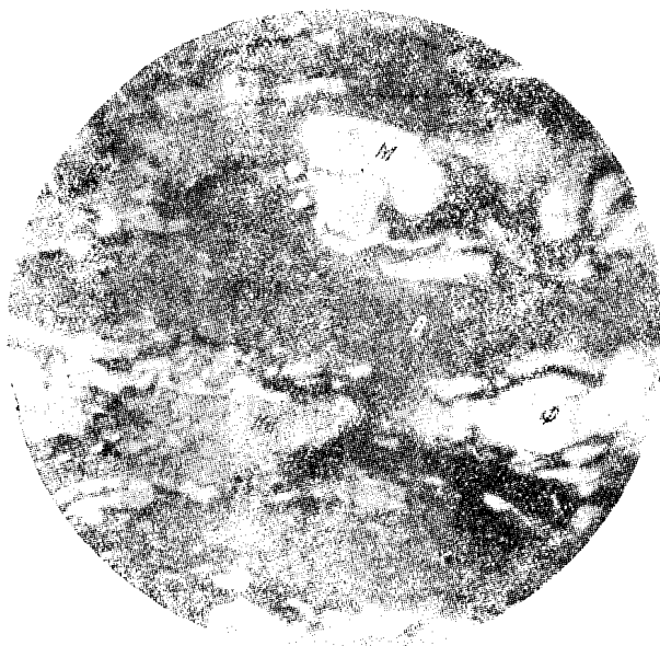
图1. 放大600倍的烟煤(庫茲巴斯)的显微结构 (И. И. Аммосов) B——鏡煤質, KB——半鏡煤質, M——不透 明質, Φ——絲炭質。
