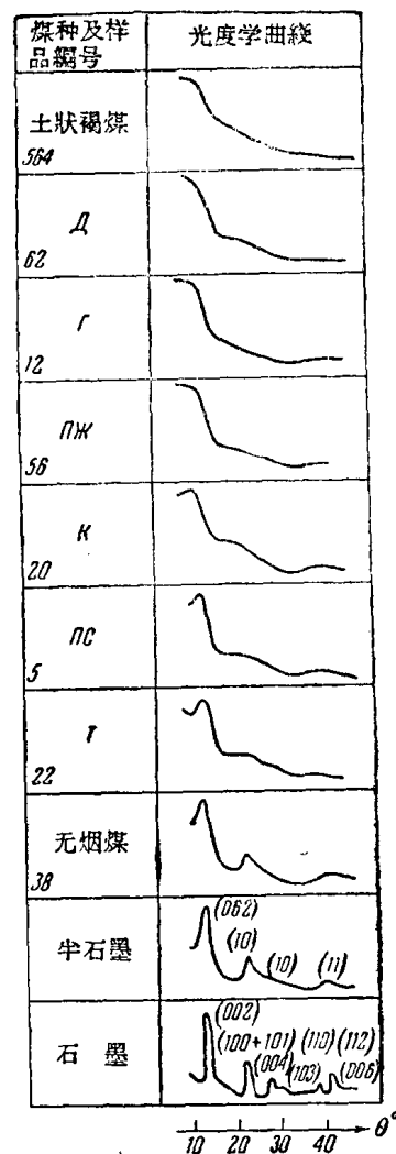
图3. 各种苏联煤和石墨 X 射线 图譜光度测定时得到的显微光度 学曲线(В. И. Касаточкин)
