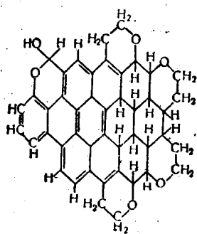
(II) C_{45}H_{36}O_8
