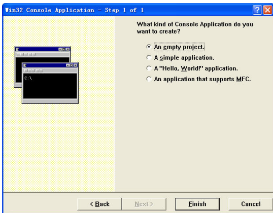
图 1-16 应用界面
