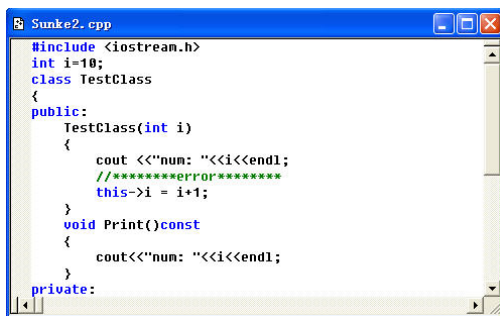
图 1-11 编辑窗口
