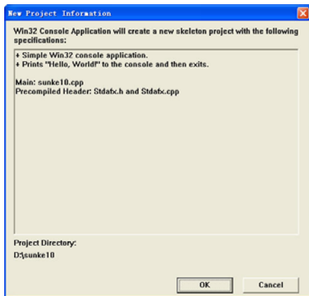
图 1-17 系统信息
