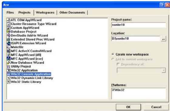
图 1-15 New 对话框
