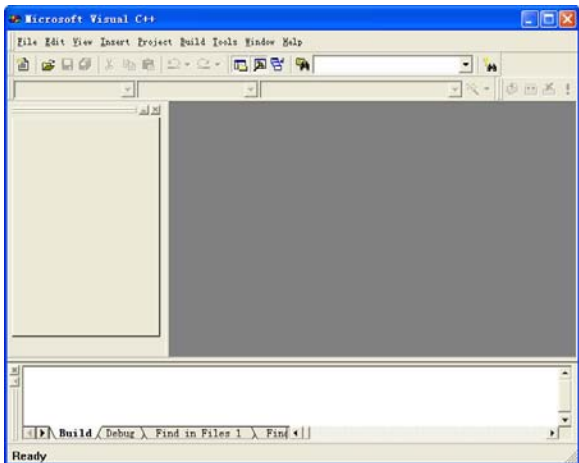
图 1-14 主窗口
