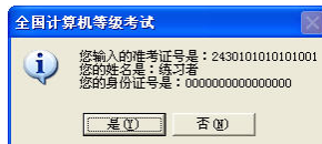
图 1-3 验证信息
