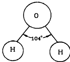
图 1-1 水分子结构
