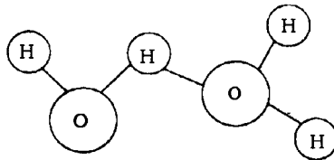
图 1-2 水分子的缔合
