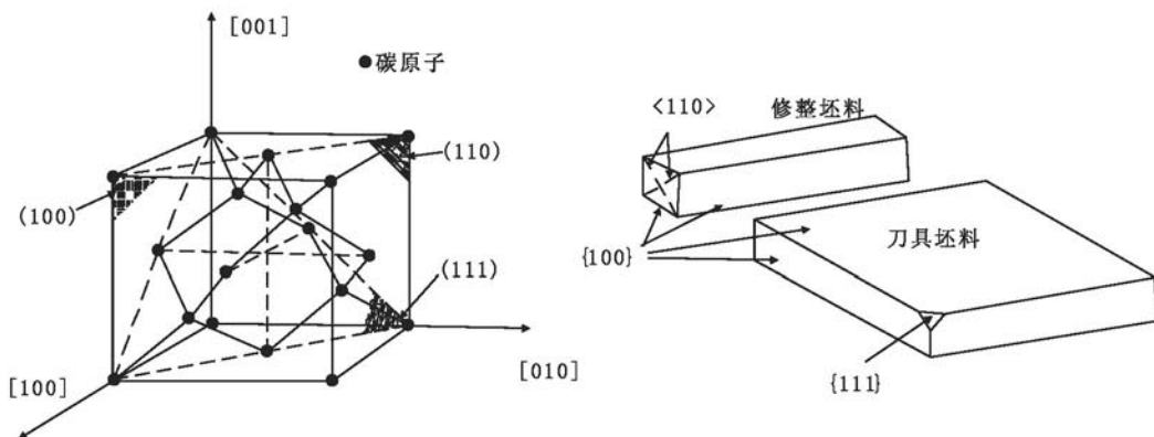
图1-3 金刚石晶体结构(左)和单晶金刚石工具坯料理想形状(右)
