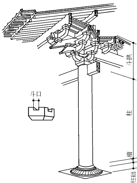
图1-1 木斗拱结构
