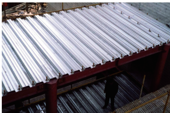
(b) 钢板压制成型后刚度可适应楼板施工要求
