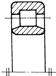
图1 滚动轴承的剖面线画法
