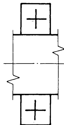
图4 绘制在轴两侧的通用画法
