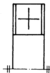
图 8 两面带密封圈的通用画法
