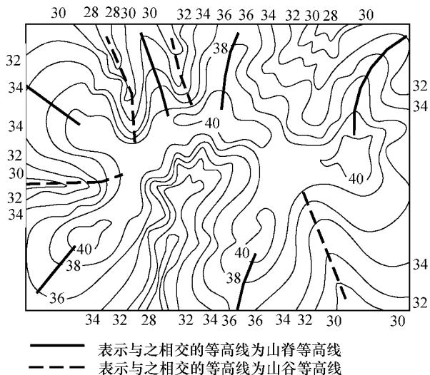
图 1-5 山脊和山谷的等高线表示图
