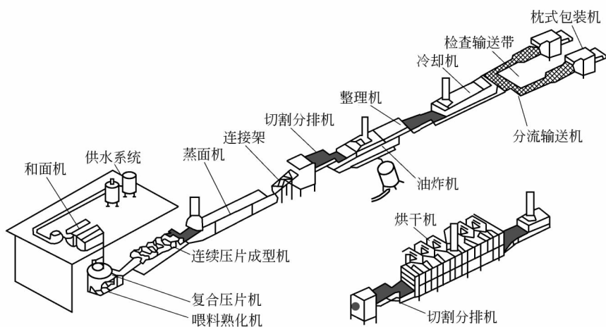
图 1-2 方便面生产工艺流程示意图
