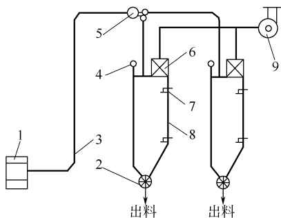
图 1-3 吸送式气力输送装置
