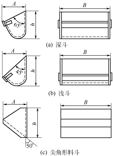
图 1-9 料斗的形式
