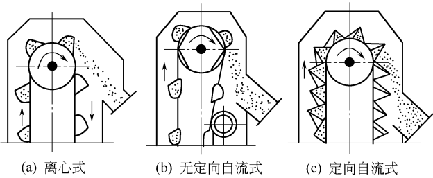
图 1-8 斗式提升机卸料方法简图
