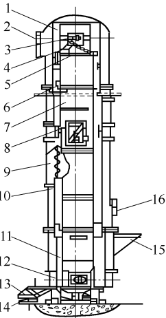
图 1-7 斗式提升机结构
