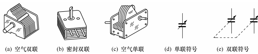
图 1.6 可变电容器的外形及图形符号
