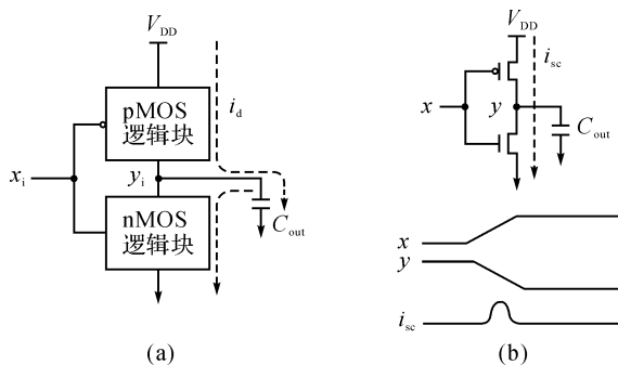
图 1.1 CMOS 门结构及其功耗分析
