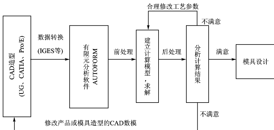
图 1.2 板料成形过程分析的流程
