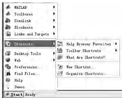
图 1-2 Start 菜单
