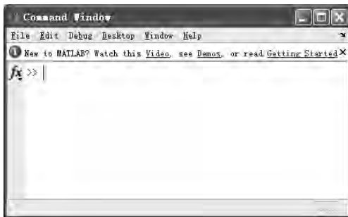
图 1-3 命令窗口
