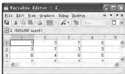
图 1-6 数组编辑器
