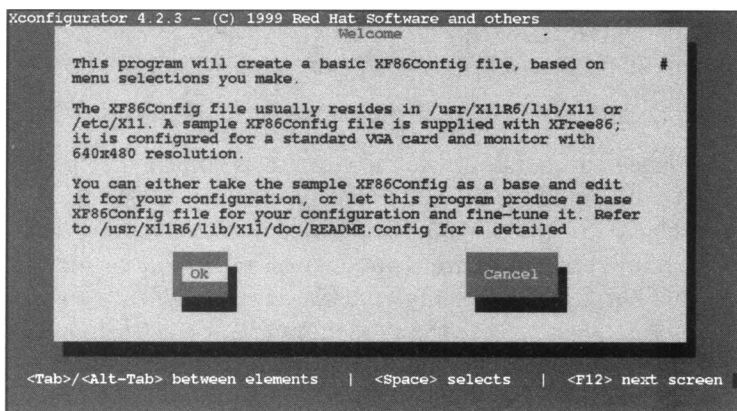
图6-11 Xconfigurator程序的初始画面
