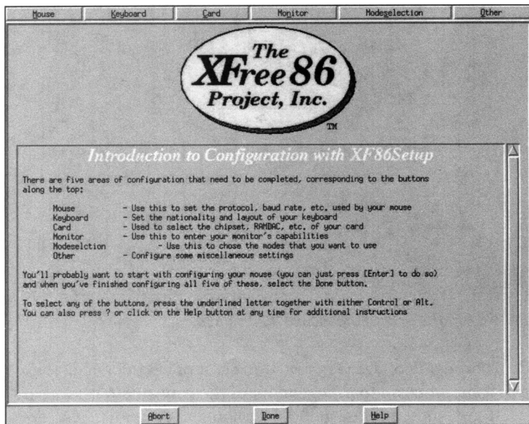
图6-3 XF86Setup程序本身
