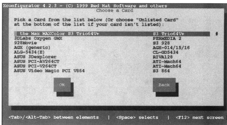
图6-12 Xconfigurator程序的图形卡选择画面
