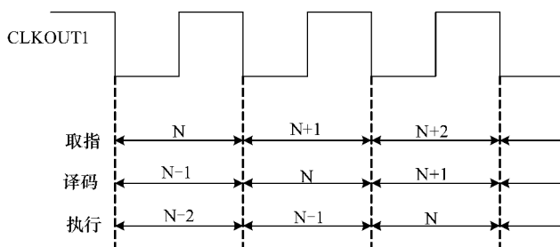
图 1-1 三级流水线操作
