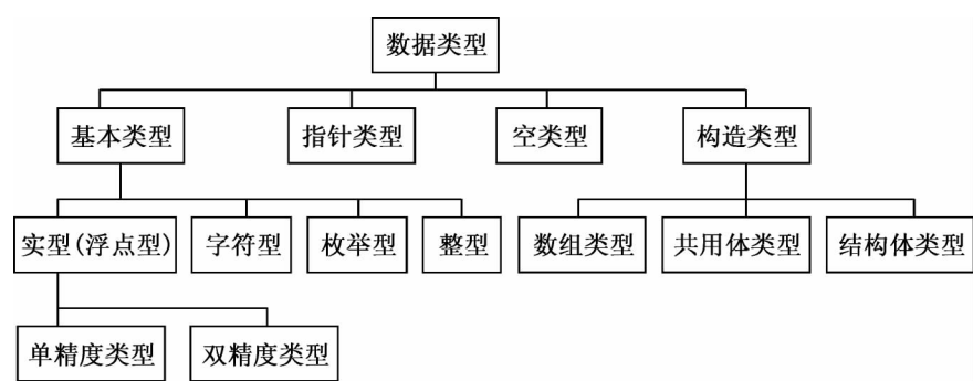
图 2-1 C 语言的数据类型
