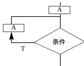
图1-8 do-while 型循环转换为 while 型循环
