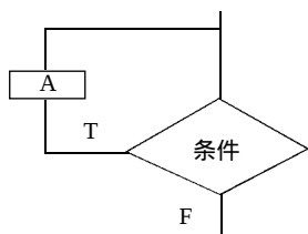
图1-6 while 型循环流程图
