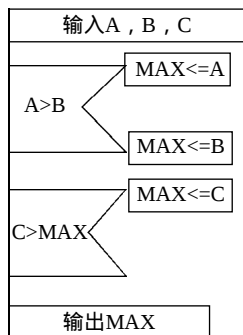
图1-18 例1-1的PAD
