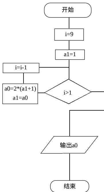
图1-3 例1-2的算法流程图
