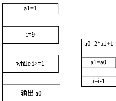
图1-19 例1-2的PAD
