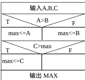
图1-13 例1-1的N-S图
