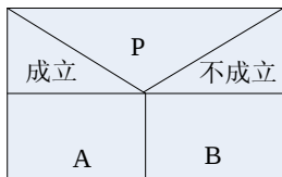
图1.9 选择结构N-S图
