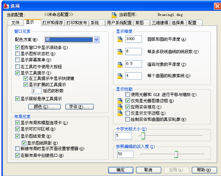
图 1.5 “选项”对话框
