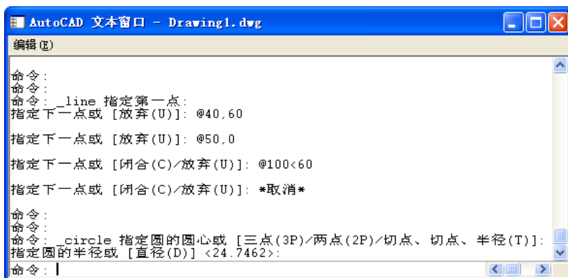
图 1.6 命令窗口
