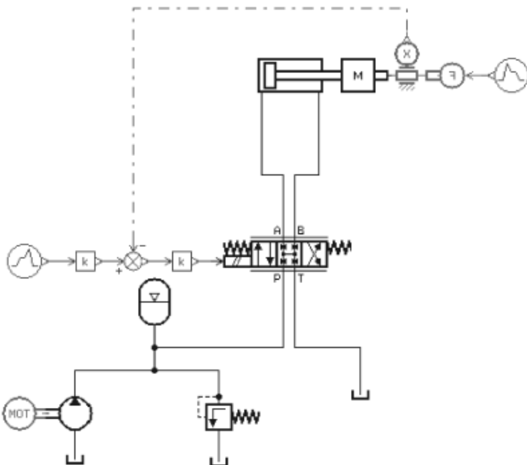
图 1.1 使用 AMESim 图标的工程系统模型
