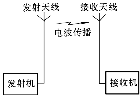
图 1 - 1 无线通信组成框图
