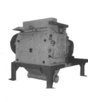
QFJ 纤 维 （ 精 制 棉 ） 专 用 粉 碎 机
