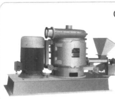
GJF 干 燥 超 微 粉 碎 机
