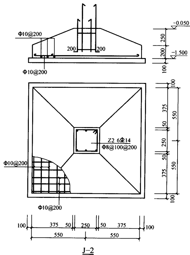
图 1.1-4 基础 J2 剖面大样
