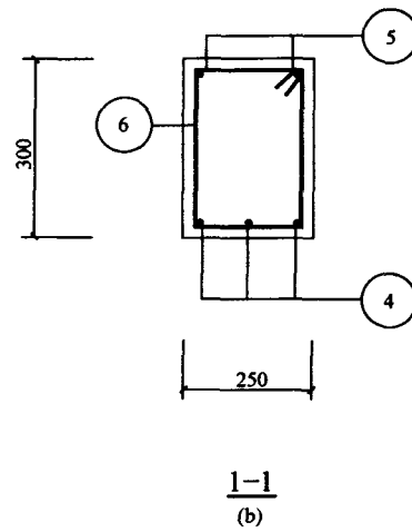
图 1.2-2 某一层结构顶板详图 (一)
