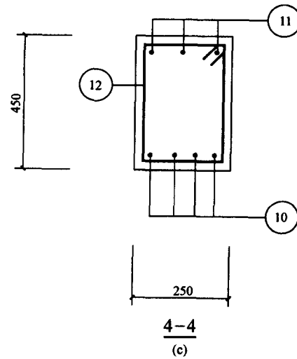
图 1.2-3 某一层结构顶板详图 (二)
