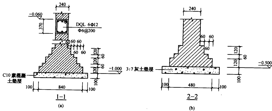
图 1.1-2 基础剖面大样
