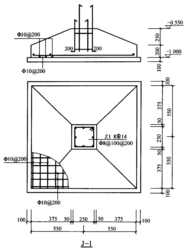
图 1.1-3 基础 J1 剖面大样
