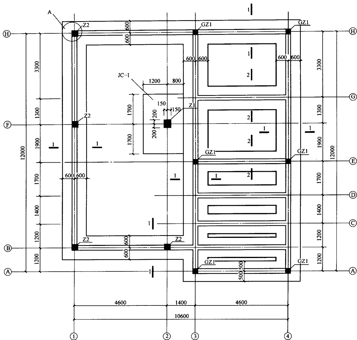
图 2.1-1 某三层结构基础布置平面
