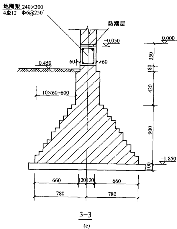
图 1.1-8 基础剖面大样
