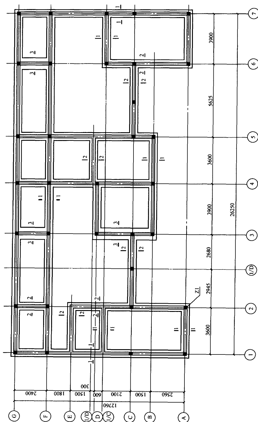
图 1.1-5 某二层结构基础平面布置图
