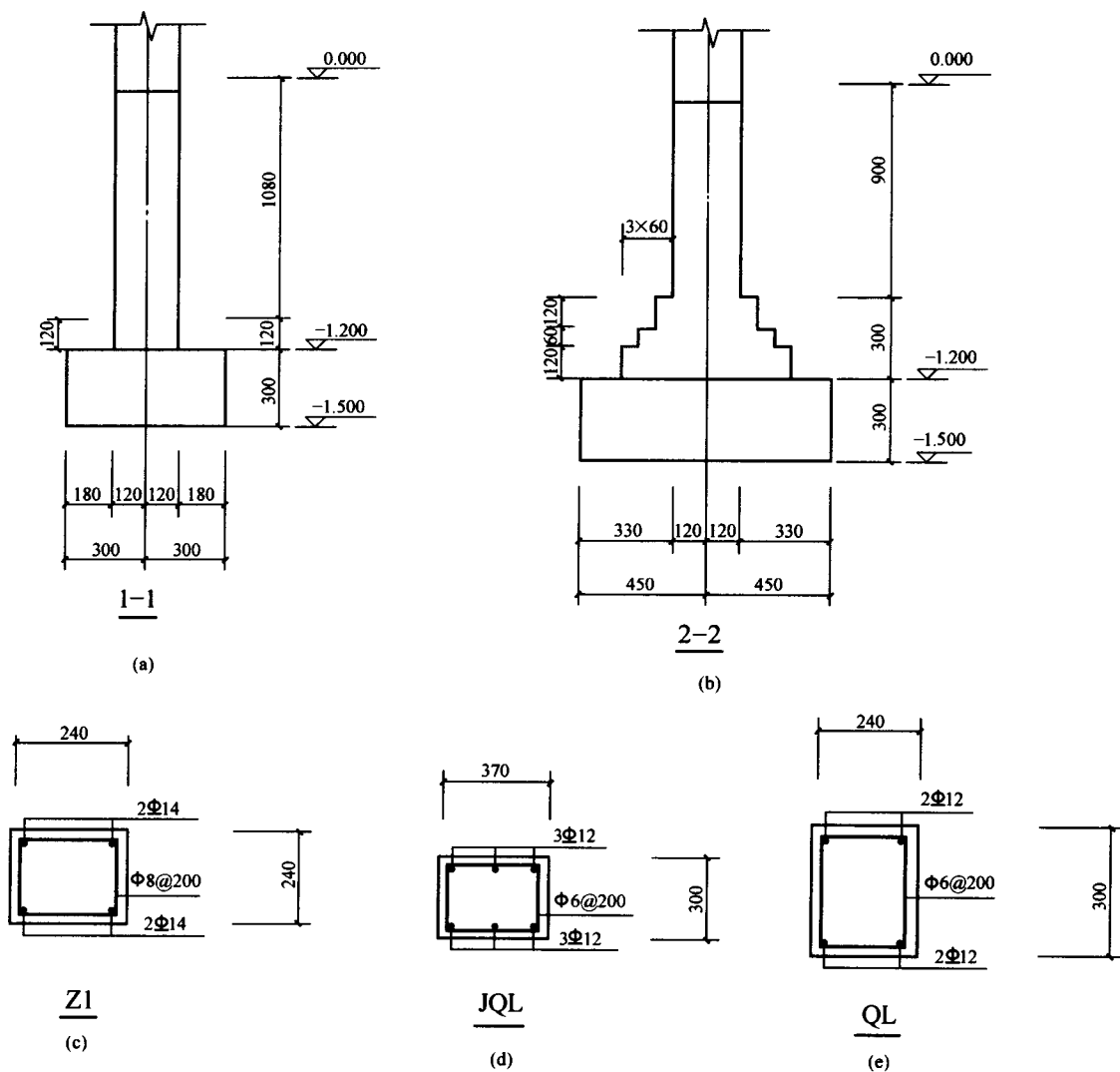
图 1.1-6 基础剖面大样
