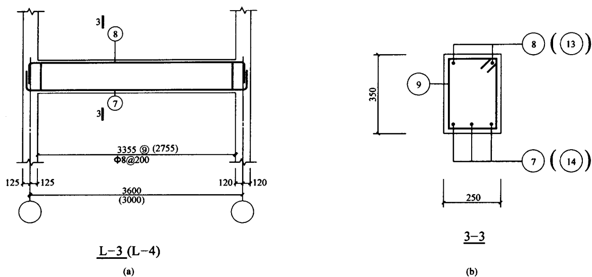
图 1.2-4 某一层结构顶板详图 (三)
