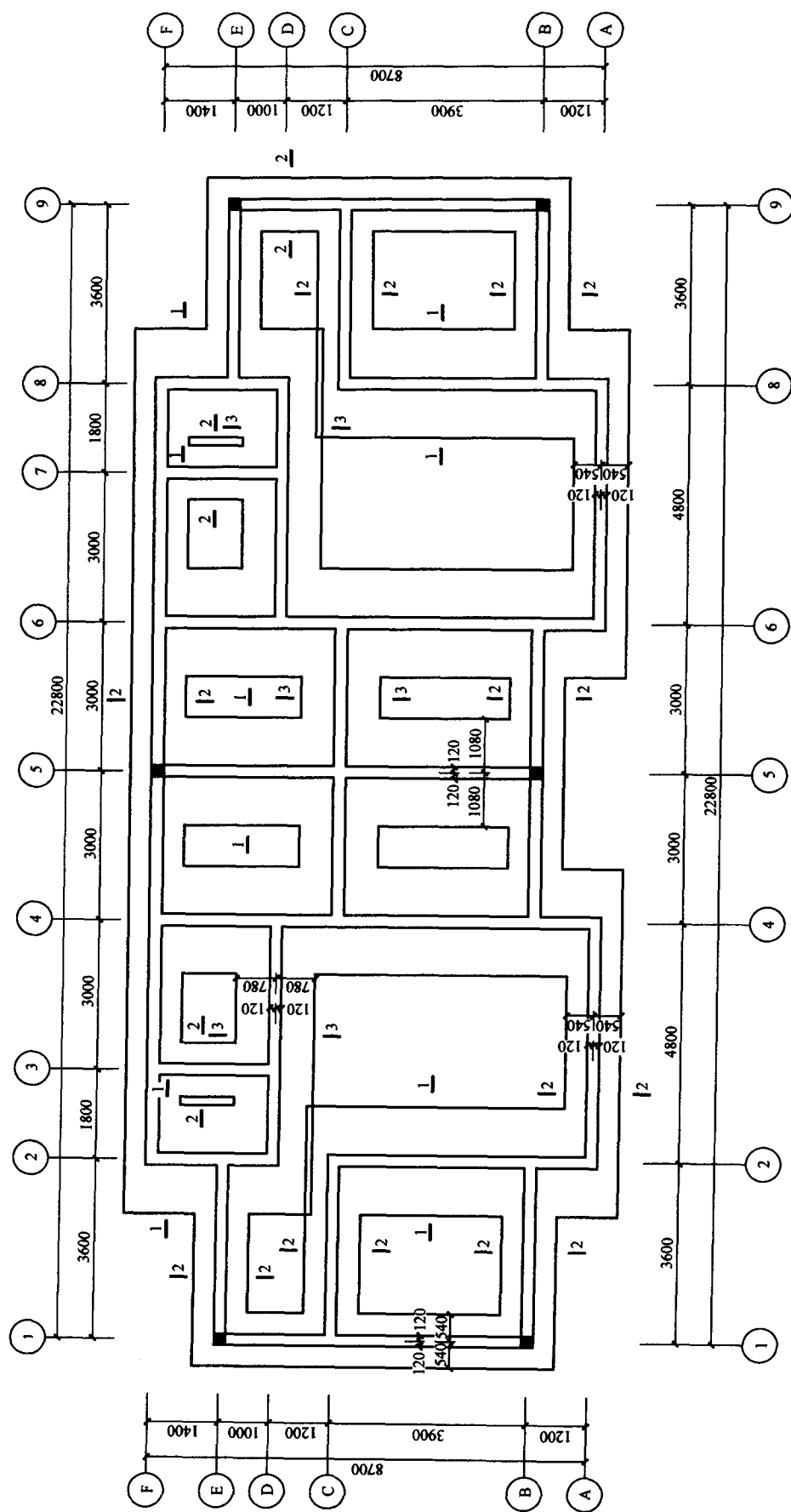
图 1.1-7 某二层结构基础平面布置图
