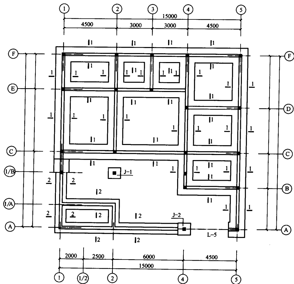
图 1.1-1 某单层结构基础平面布置图
