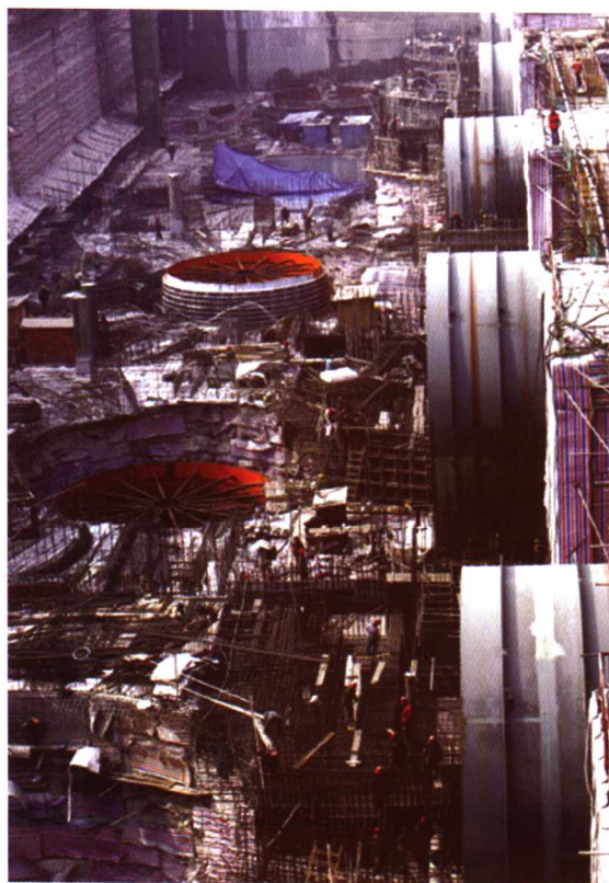
三峡水电站右岸厂房建设
