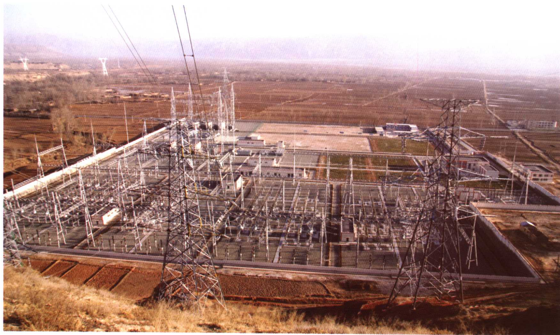
750kV 官亭变电站
