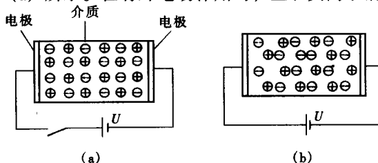
图 1-2 离子式极化示意图
