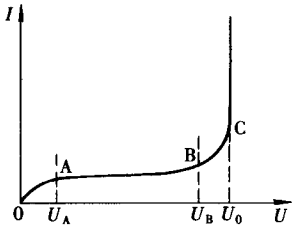
图 1-6 气体电介质中的电流和外施电压的关系
