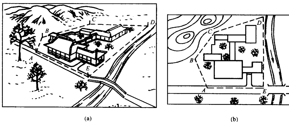
图 1-9 测量地形平面图的方法
