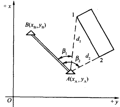
图 1-6 确定平面上点位的原理
