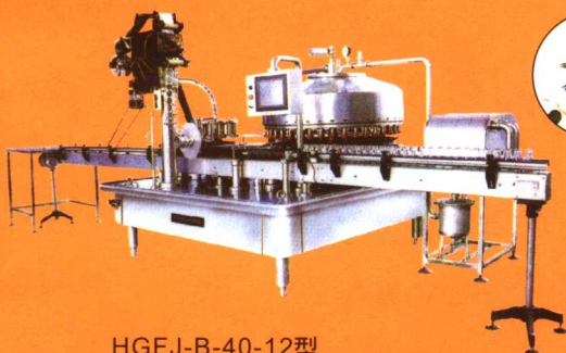
HGFJ-B-40-12型 回转式全自动玻璃瓶灌装封口机
