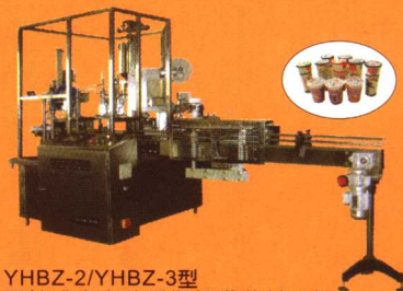
YHBZ-2/YHBZ-3型 回转式全自动纸塑杯灌装封口机
