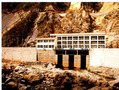
建设中的文泾水电站主厂房
