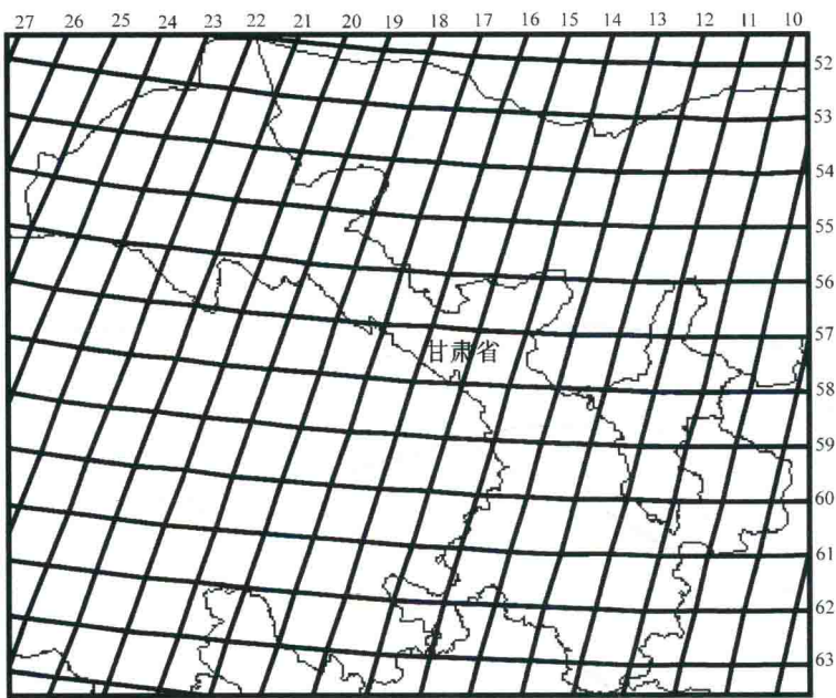
图1-1 甘肃省CBERS影像覆盖示意图
