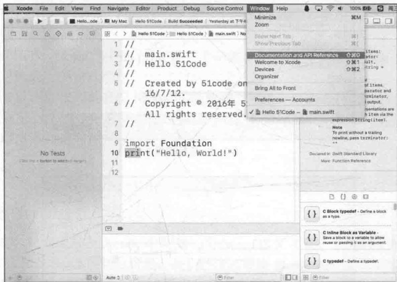
图 1-7 查找 API
