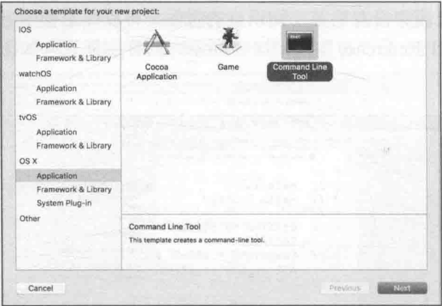
图 1-8 选择模板
