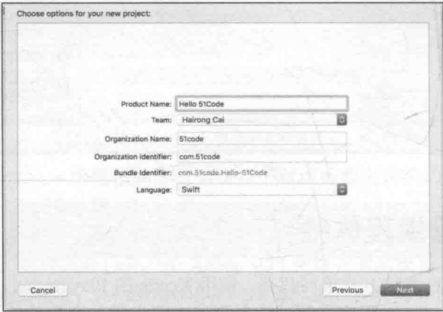
图 1-9 填写信息
