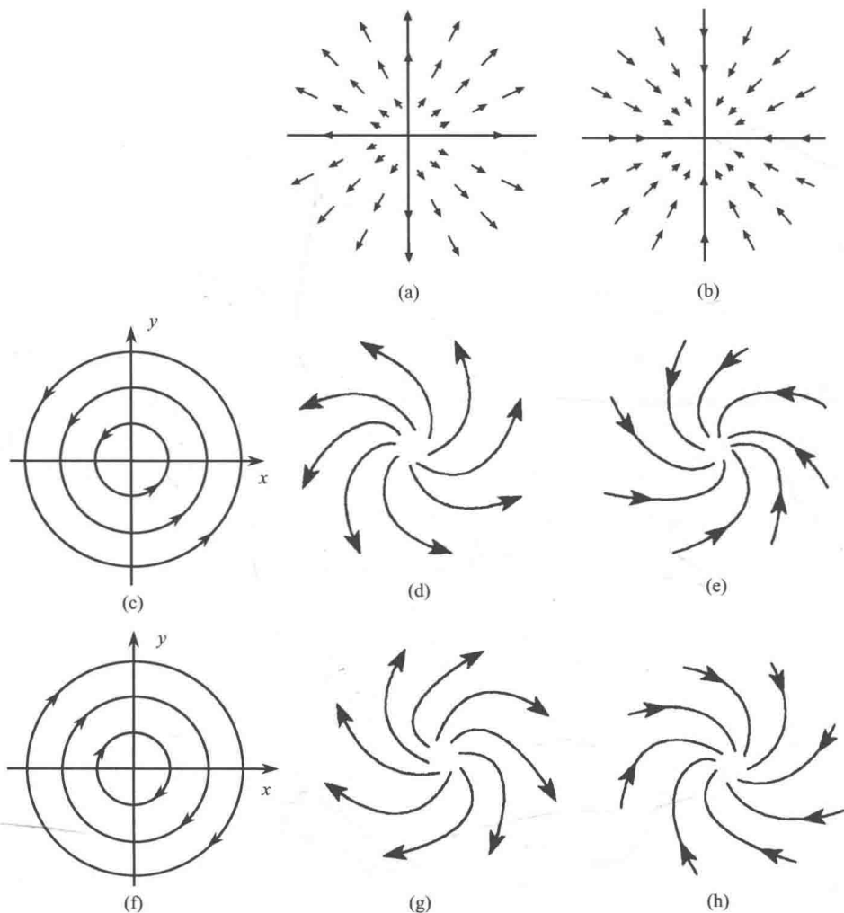
图 1.7 涡旋以及流入(汇)和流出(源)流型
