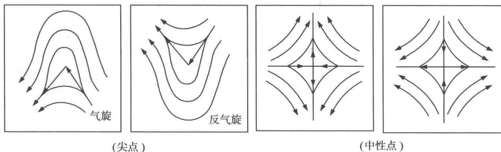
图 1.6 尖点和中性点
