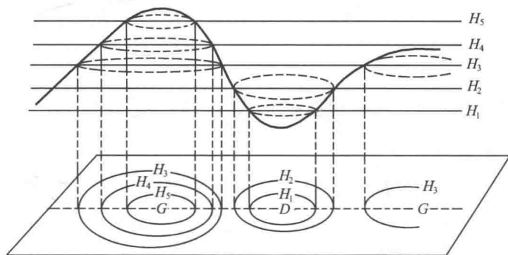
图 1.3 等压面(粗线)和等高线(虚线)
