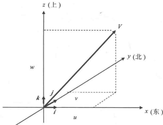
图 1.8 三维风矢量的 u, v, w 分量
