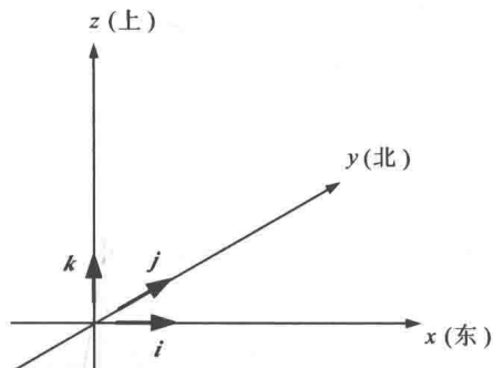
图 1.2 z 坐标系
