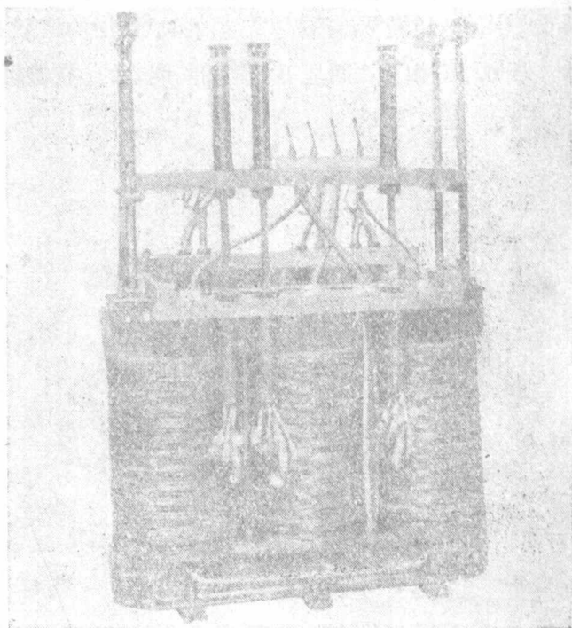
圖 7. 3 相變壓器的鐵心和繞組。
