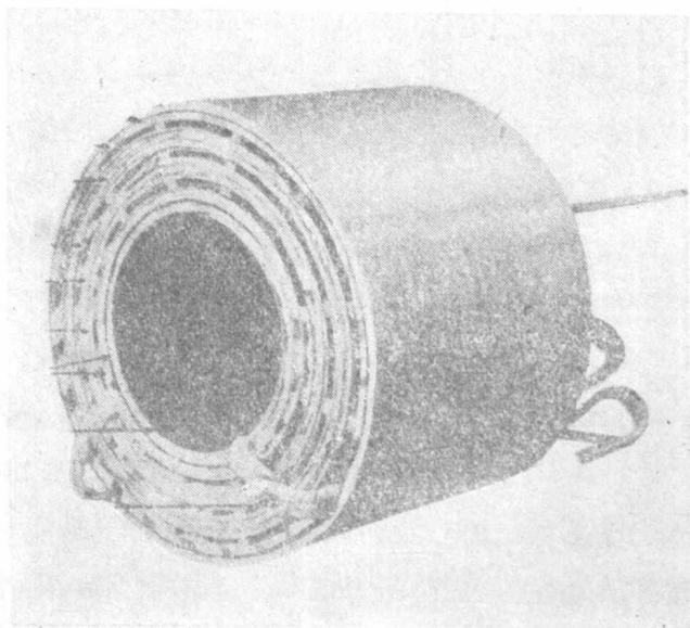
圖 6. 分層的變壓器繞組。
