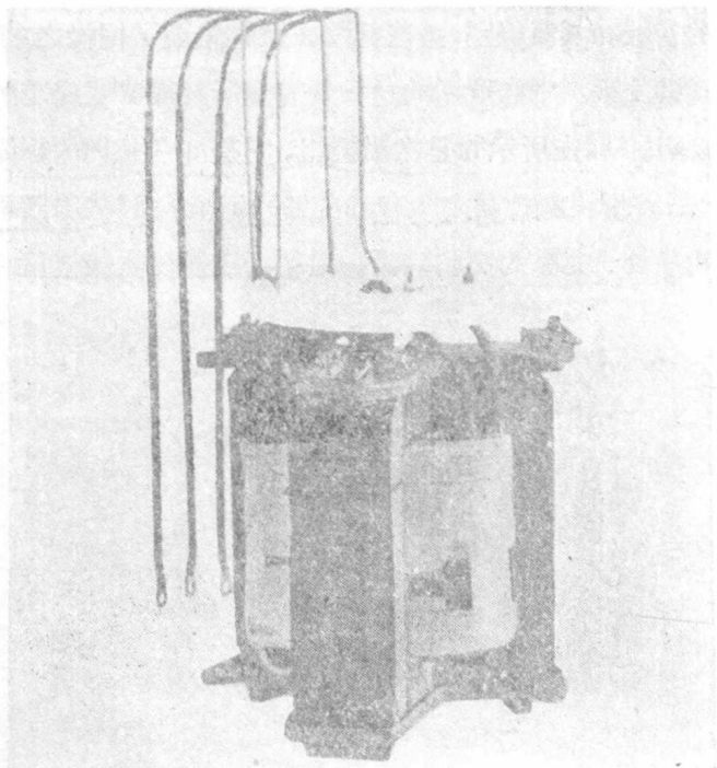
圖 5. 完整的變壓器鐵心和繞組。
