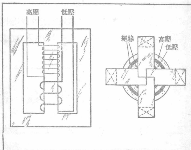
圖 2. 外鐵式變壓器。
