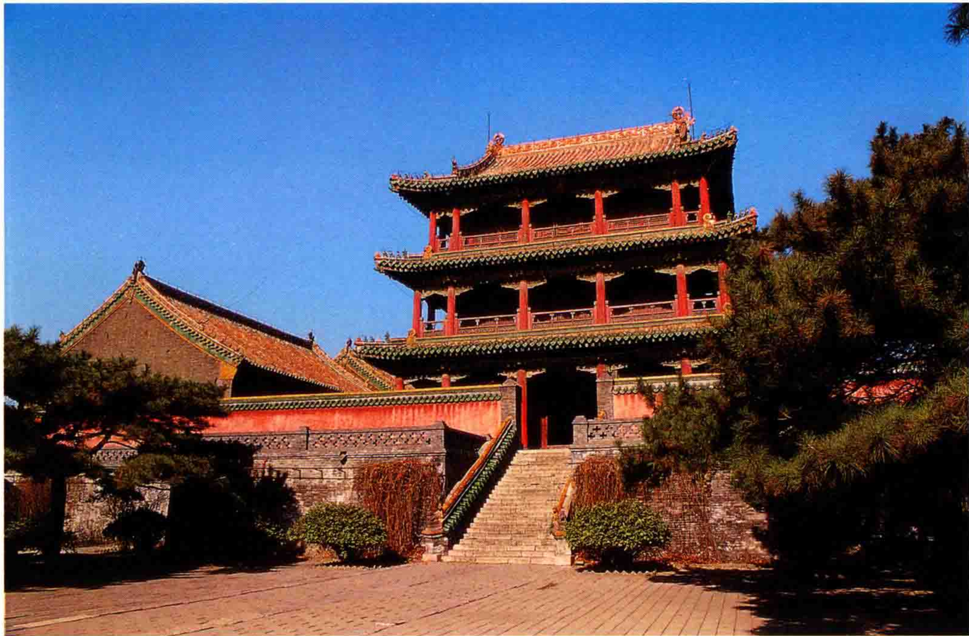
图1-2 辽宁沈阳故宫凤凰楼（覃力 摄）
