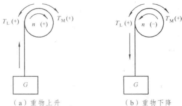
图 2.2 电动机拖动重物升降
