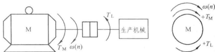
图 2.1 单轴旋转拖动系统
