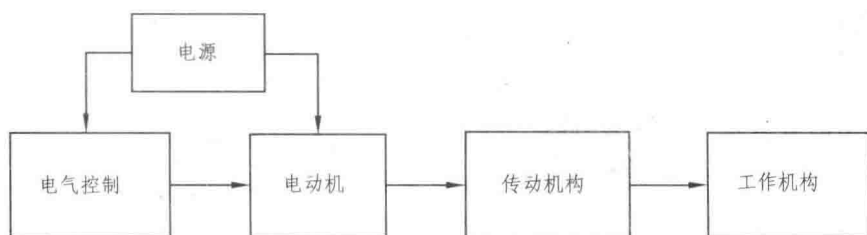
图 1.1 机电传动系统组成
