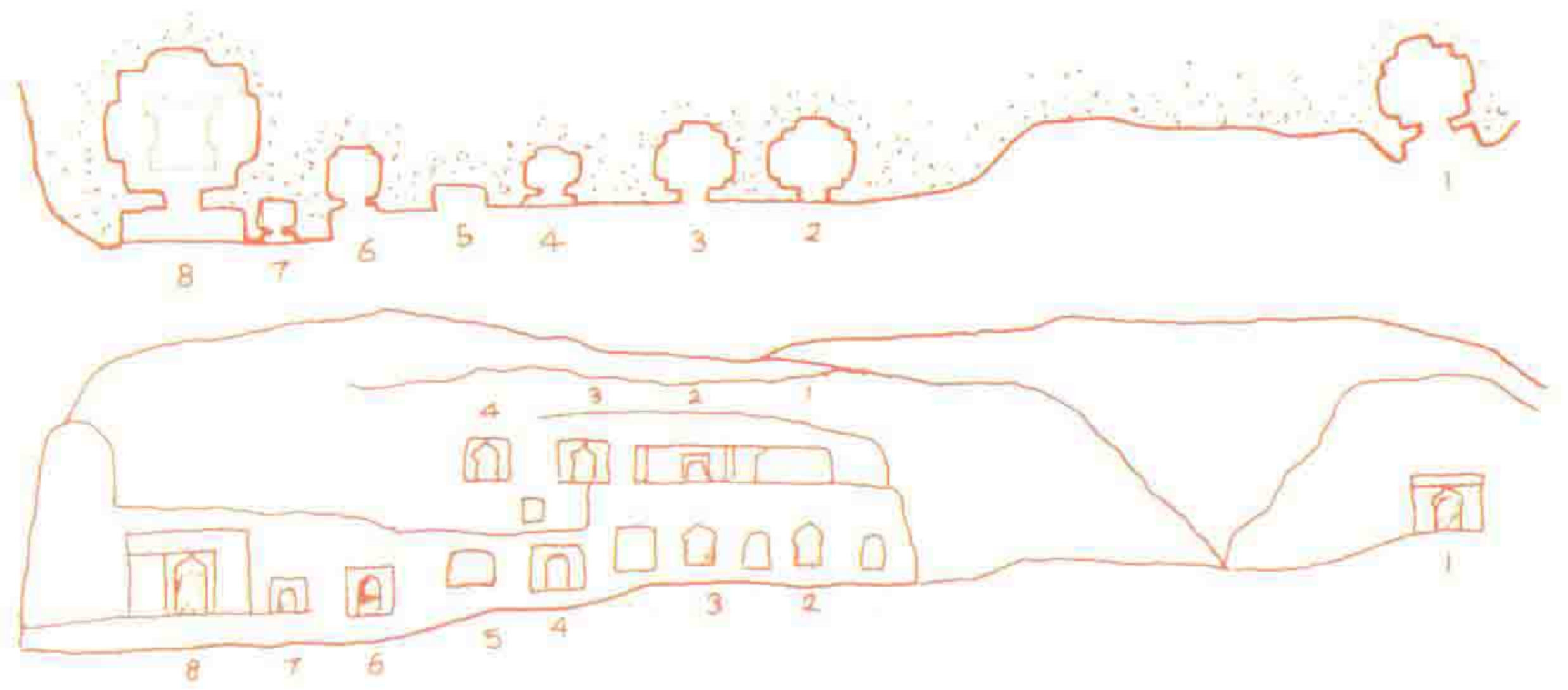
图1-2 天龙山东峰洞窟平面图和立面图（示意图）
