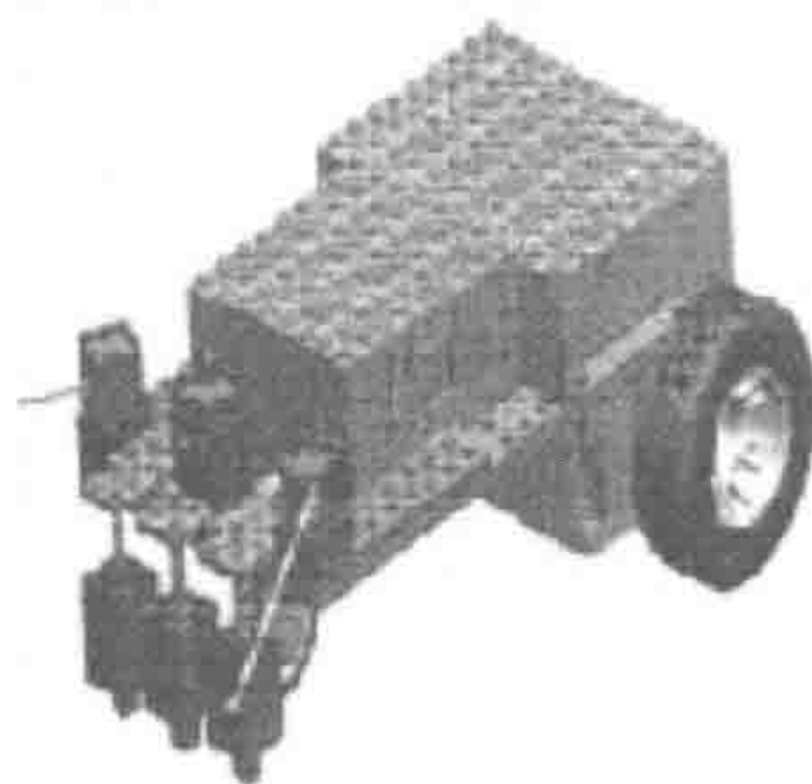
图 1-9 中鸣简易版 积木机器人套件
