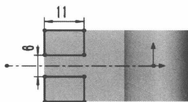
图 1.6 横断面草图
