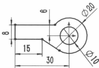
图 1.3 横断面草图
