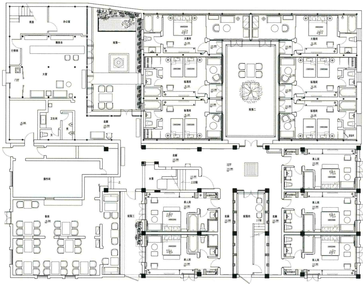
一层平面图
