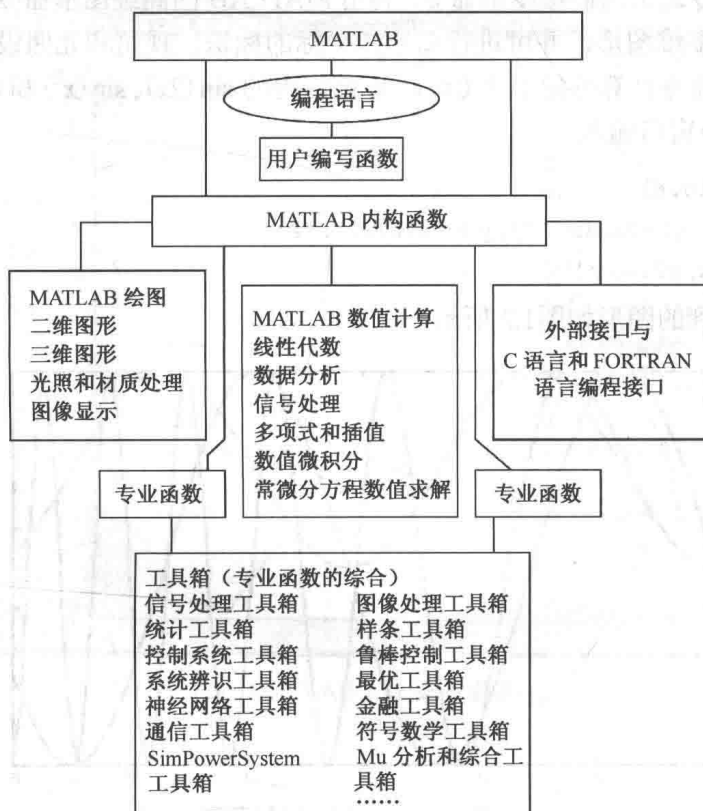
图 1.1 MATLAB 的主要结构和功能
