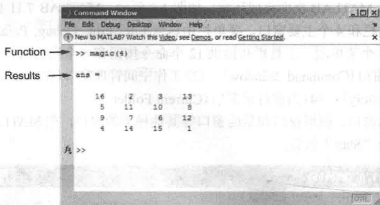
图 1.4 MATLAB 命令窗口
