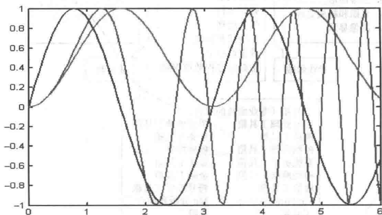
图 1.2 函数 \sin(2x) , \sin(x^2) 和 (\sin(x))^2 的图形
