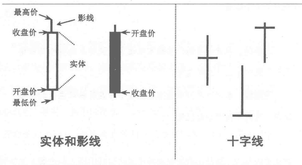
图 1-4 K 线图的构成
